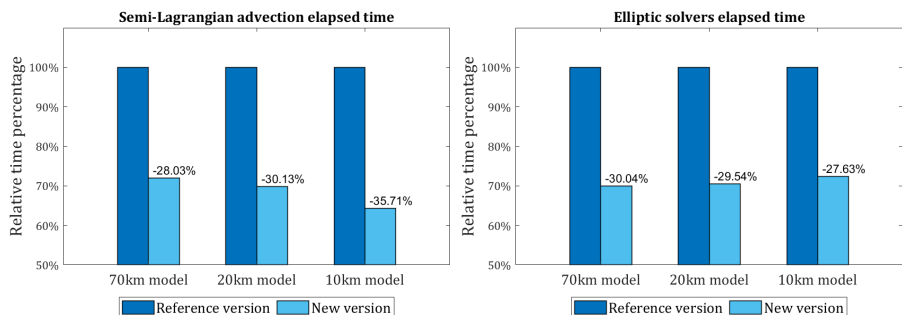
Рис. 6 — Изменение времени расчетов в блоках полулагранжевой адвекции (слева) и решении эллиптических уравнений (справа) для модели ПЛАВ с разрешением 10, 20 и 70 км в результате внедрения одинарной точности.
