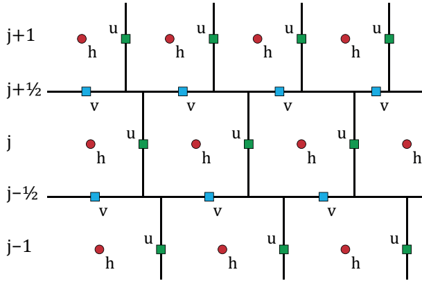
Рис. 1 — Схематичное изображение расположения узлов редуцированной широтно-долготной сетки с разнесением переменным.
