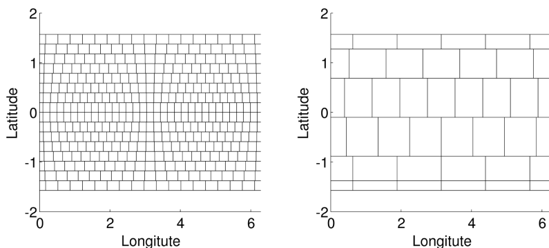
Рис. 2 — Пример применения двух итераций предложенного алгоритма условного сгрубления для редуцированной широтно-долготной сетки.
