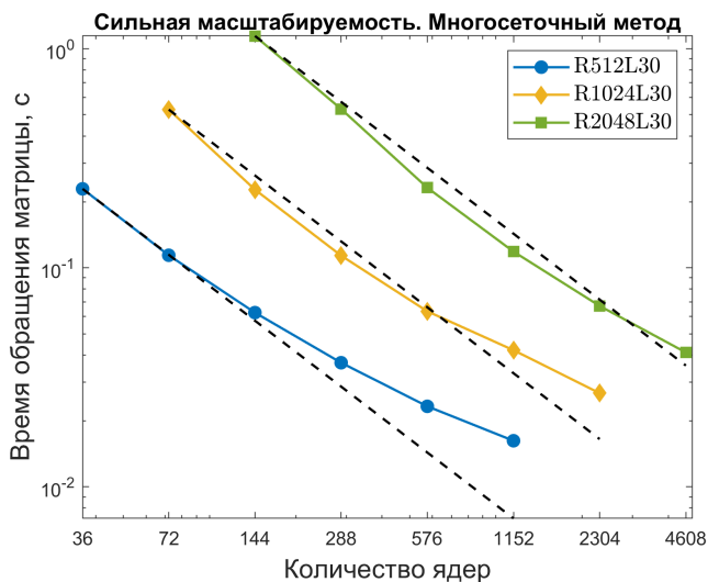
Рис. 3 — Сильная масштабируемость многосеточного алгоритма. Число после R в обозначении сетки — количество узлов сетки вдоль долготы на экваторе, число после L — число вертикальных уровней расчетной сетки.
