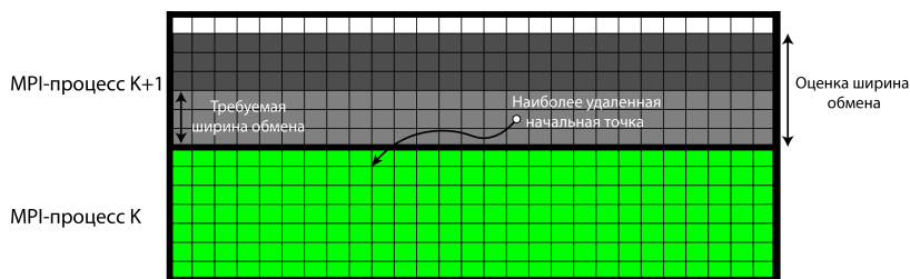
Рис. 4 — Область параллельной зависимости в полулагранжевом блоке. Априорная оценка — темно-серый цвет, оценка, основанная на положении начальных точки полулагранжевых траекторий — серый цвет.
