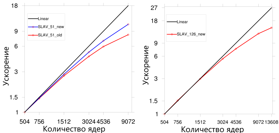
Рис. 5 — Сильная масштабируемость кода модели ПЛАВ. Левый рисунок – сравнение версий с фиксированной (красная линия) и адаптируемой (синия линия) шириной обмена на сетке 3024 \times 1513 \times 51 . Правый рисунок – версия с адаптируемой шириной обмена на сетке 3024 \times 1513 \times 126 .
